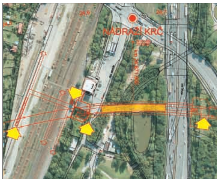
STANICE NÁDRAŽÍ KRČ – Povrchová stanice se dvěma vestibuly. Bude plně využita možnost přímého kontaktu se železniční tratí směřující na Vrané nad Vltavou a Dobříš/Čerčany a do centra Prahy. Půjde o komplexní řešení celého přestupního uzlu (rekonstrukce železniční části přestupního uzlu je závislá na finančních možnostech Správy železniční dopravní cesty). Význam přestupního místa poroste s postupným zaváděním intervalové dopravy na této železniční trati. Do koncepce řešení stanice trasy D bude zahrnuto i širší okolí.
